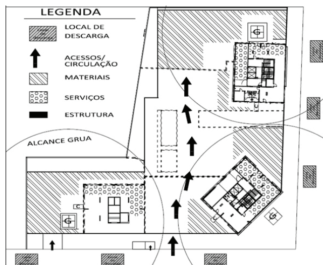
Figura 4. Croqui esquemático do layout elaborado para o canteiro de obras.
